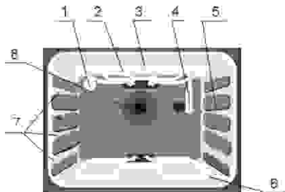
Рисунок 5.6 – Электрический жарочный шкаф
