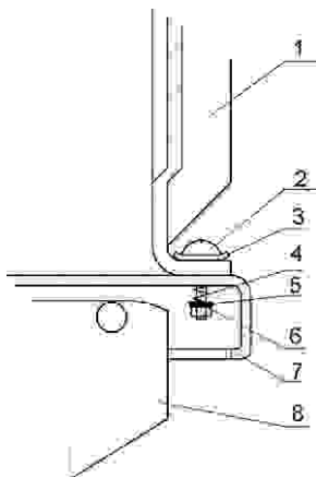
Рисунок 6.1 - Установка щитка на плиту
