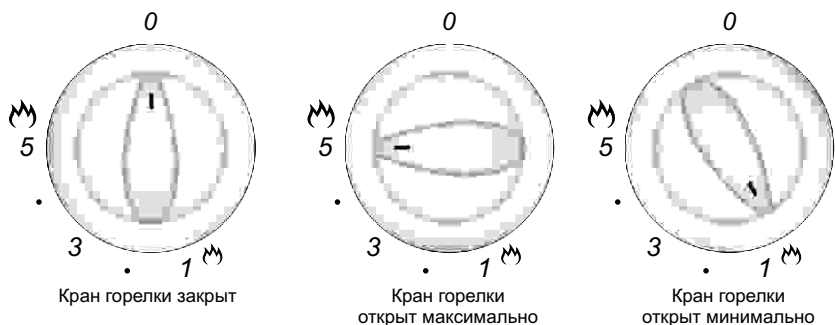
Рисунок 7.3 – Возможные положения ручки крана газового жарочного шкафа. Цифры носят ориентировочный характер.
