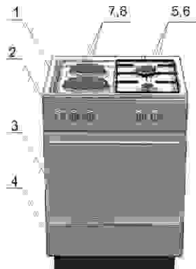
Рисунок 5.3 – Общий вид плиты (2 горелки рабочего стола, 2 чугунные конфорки)
