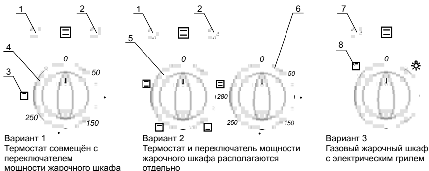
Рисунок 7.2 – Ручки управления электрическими нагревательными элементами жарочного шкафа
